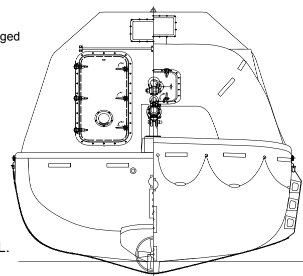
REAR/FRONT VIEW
